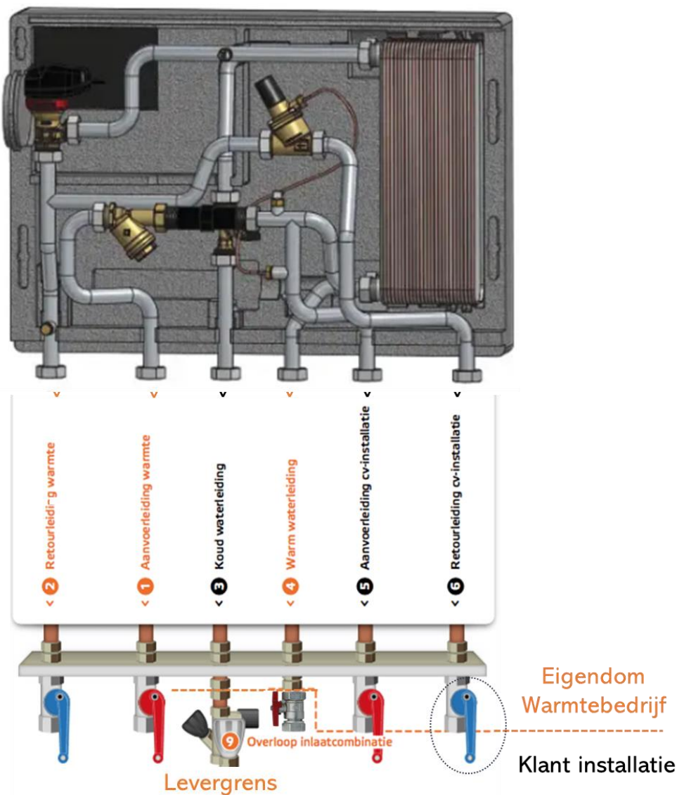
Afbelding 1: Levergrens en aansluitbeugel
